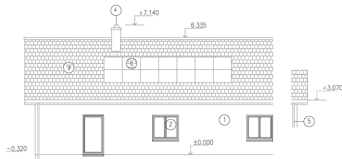
POHLED SEVEROVÝCHODNÍ
