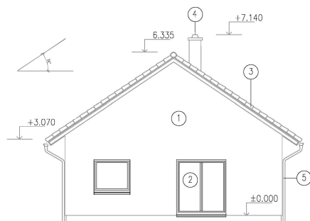
POHLED SEVEROZÁPADNÍ :
