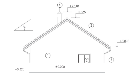
POHLED JIHOVÝCHODNÍ
